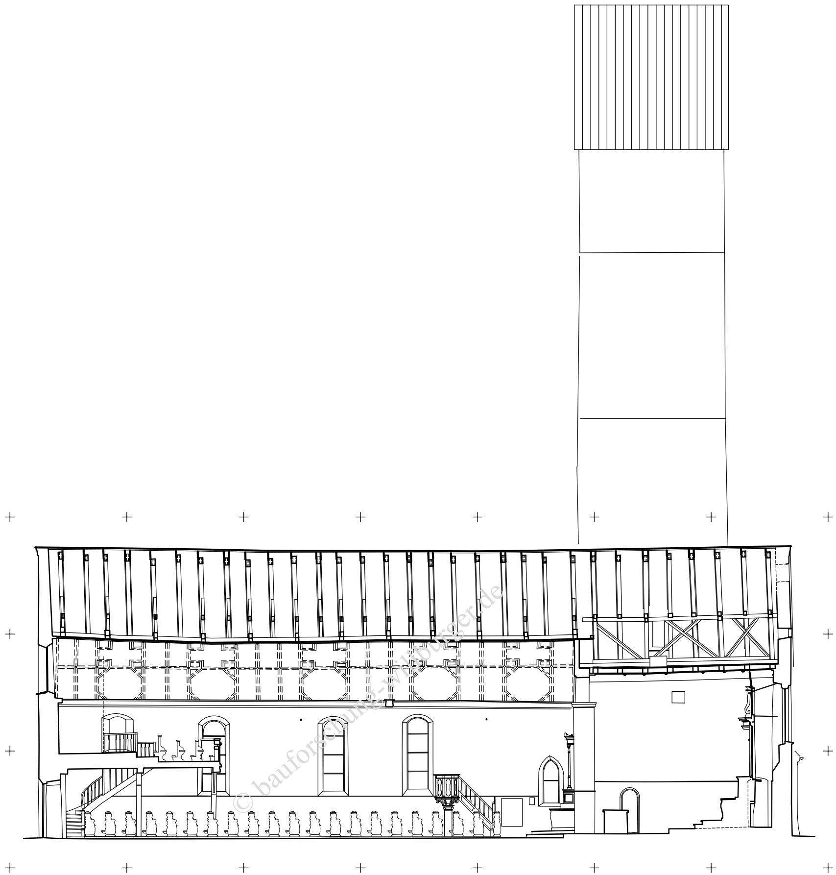
Längsschnitt
